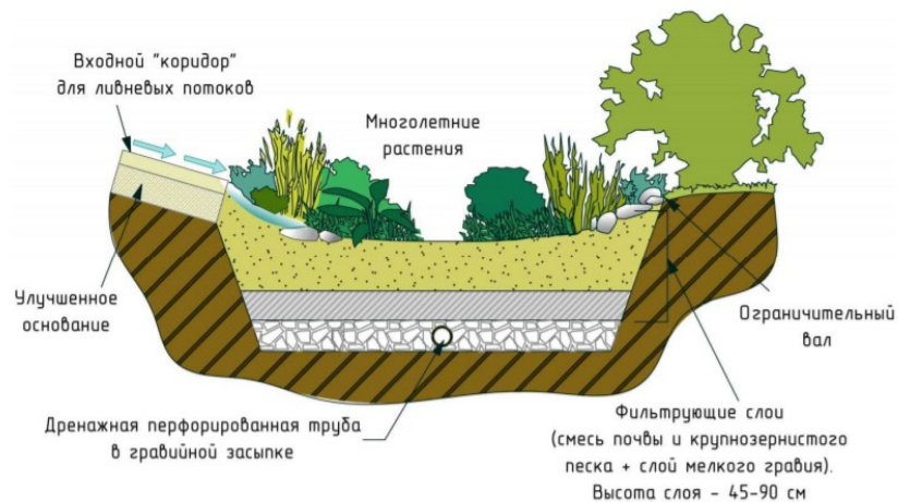
Рис. 1. Схема устройства дождевого сада
