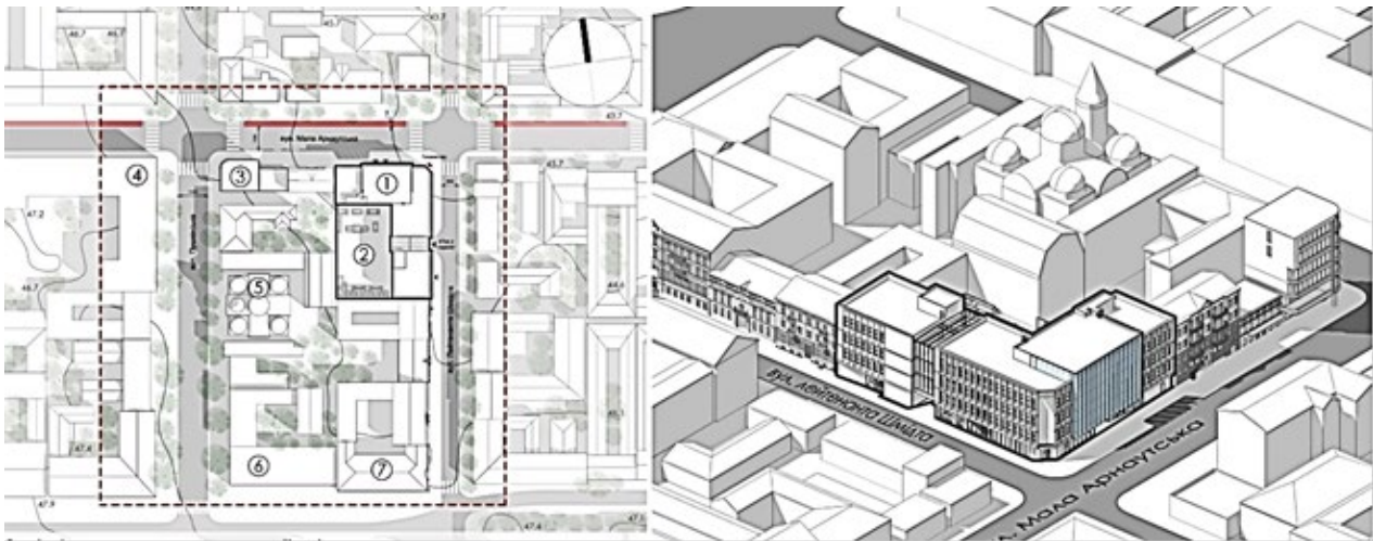
Рис. 2. Громадсько-виставковий комплекс в історичному середовищі м. Одеси. Містобудівне рішення. Пропозиції – архітектор І. Лесів
