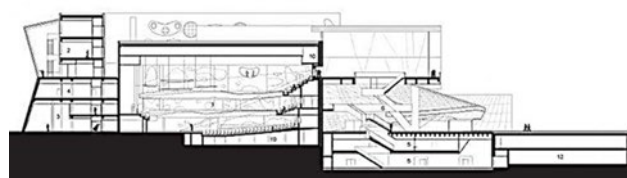
г) Поздовжній розріз по залу для глядачів
